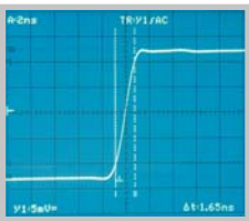
Überschwingungsarme Messverstärker
